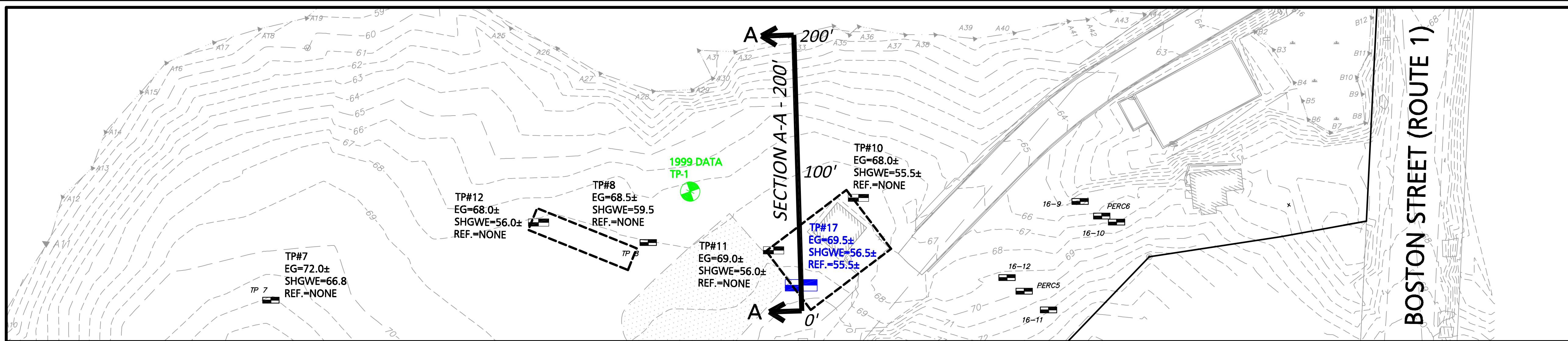
TEST PITS - PLAN VIEW N.T.S.
